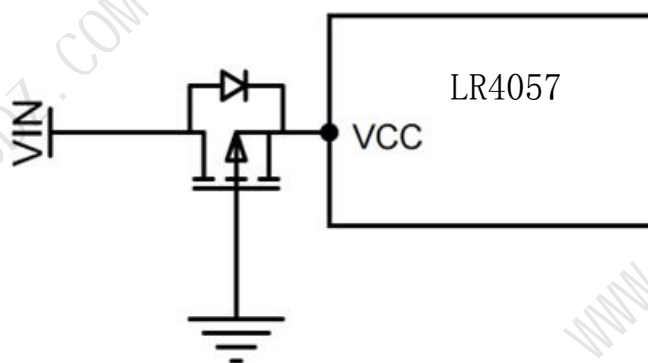
低损耗输入反向极性保护
