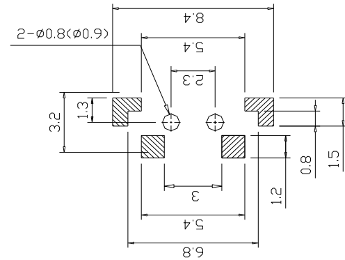
PCB. 焊接图
